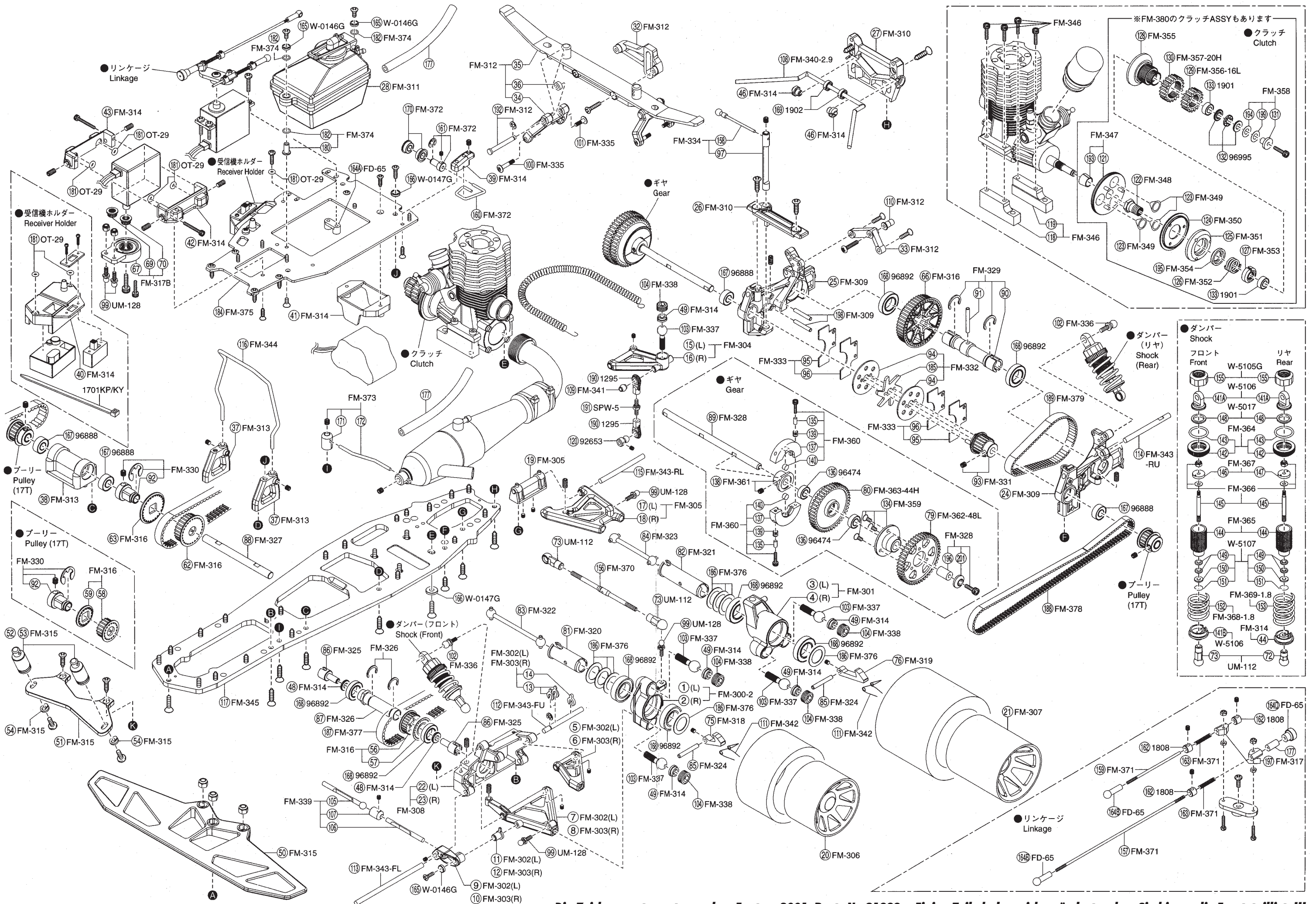
Die Zeichnung stammt vom dem Fantom 2001, Best.-Nr. 31999 • Einige Teile haben sich geändert, sehen Sie hierzu die Ersatzteilliste!!!
